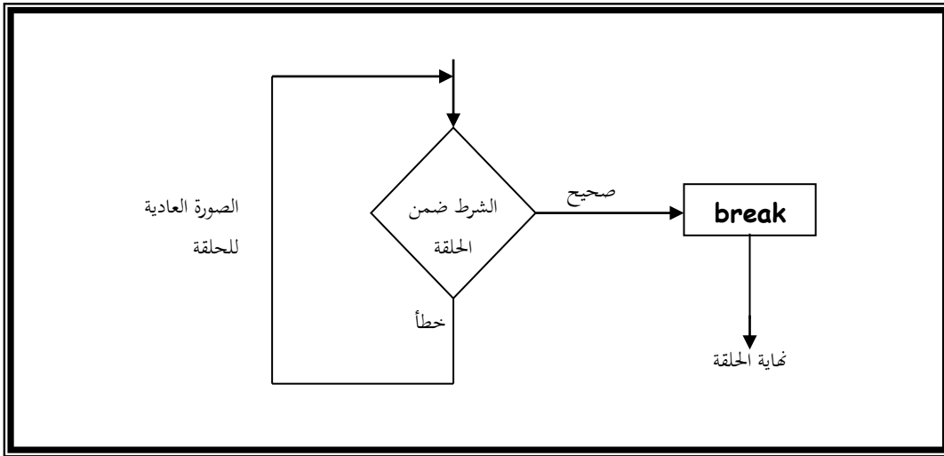
شكل (٣-٤) - طريقة عمل العبارة break
