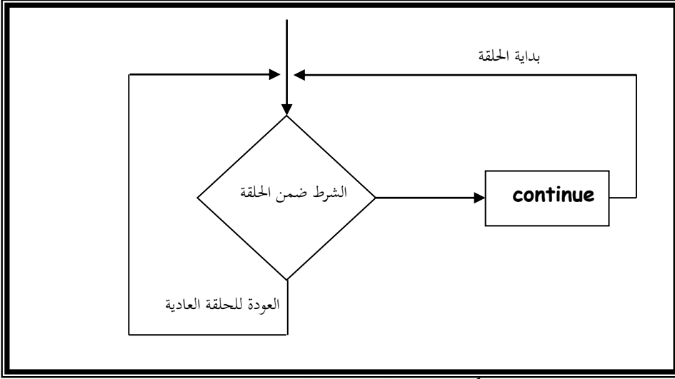
شكل (٥-٣) طريقة عمل العبارة continue
