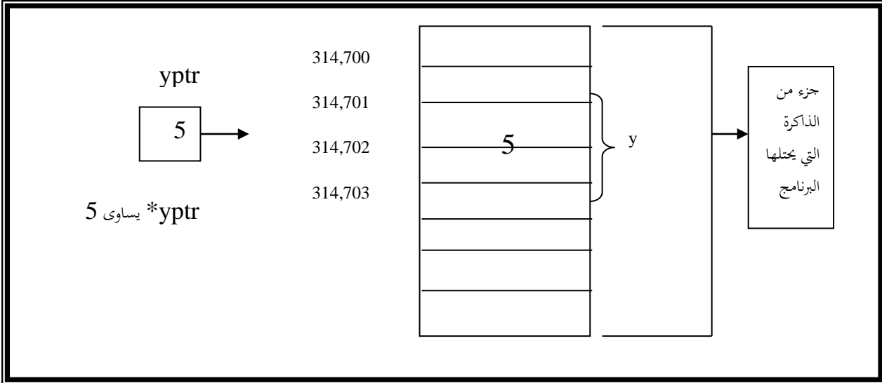
شكل (٥-١) يوضح المخرج من *yptr
