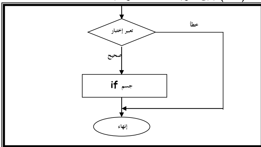
شكل (٢-١) طريقة عمل العبارة if
