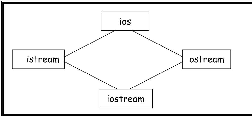
الشكل ١١-١ يوضح هرمية فئات الدفق
