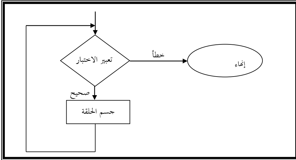
شكل (٣-١) - طريقة عمل الحلقة while
