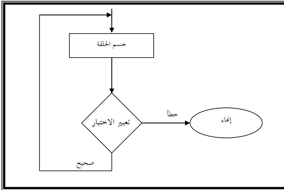
شكل (٢-٣) - طريقة عمل الحلقة do
