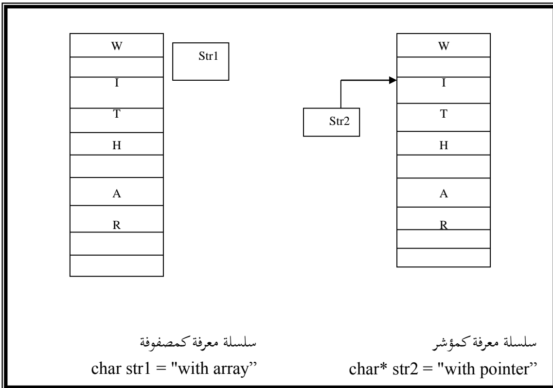
شكل (2-5) يوضح محتوى الذاكرة في حالتي التعريف كسلسلة والتعريف كمؤشر
