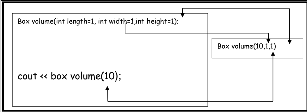
شكل (٢-٤) يوضح كيفية تزويد الوسيطات الافتراضية
