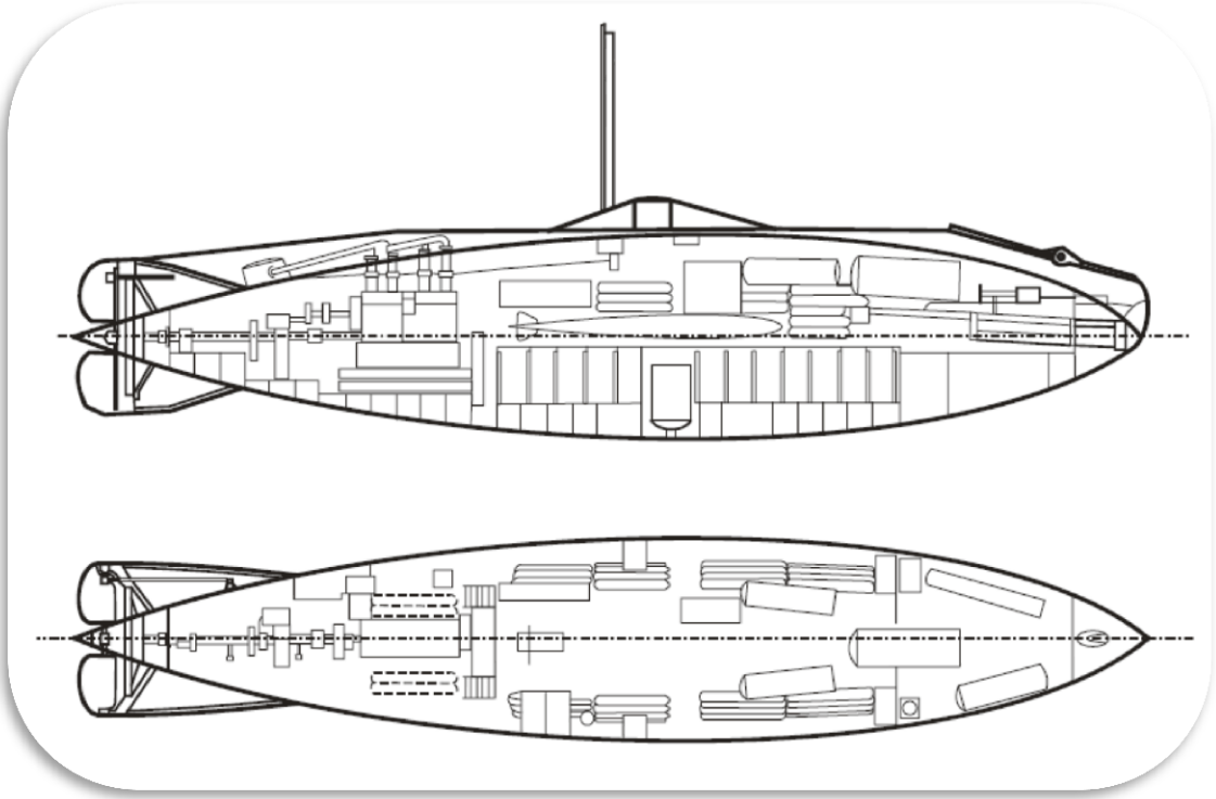
شكل ( ٢٢ ) مخطط الغواصة هولاند
