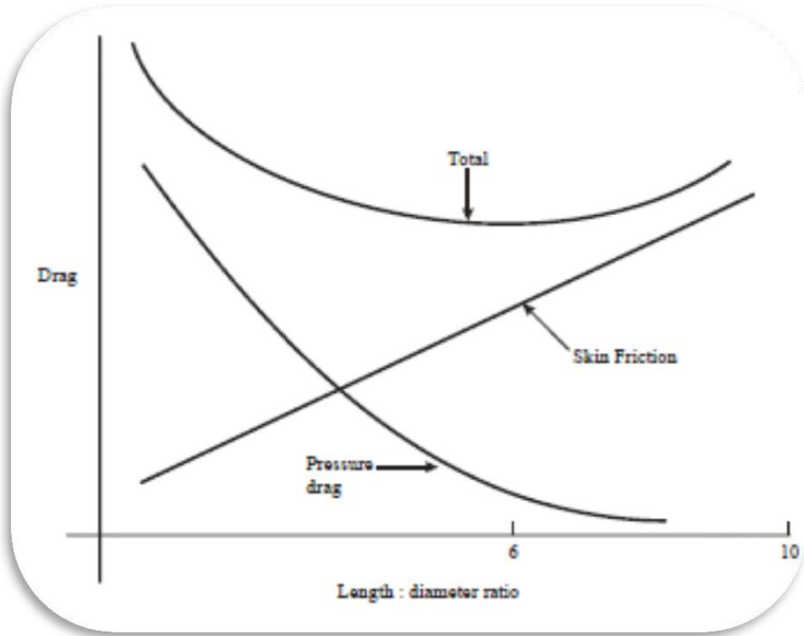
شكل ( ٥٣ ) : العلاقة بين ثابت الحجم الى الاعاقة (Drag).
