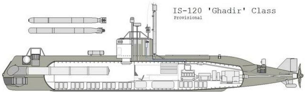
الشكل ( ٥٩ ) : مخطط الغواصة الكورية IS -120
