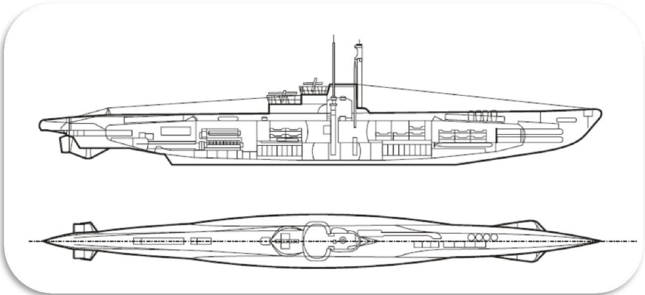
شكل ( ٢٥ ) مخطط الغواصة الألمانية نوع VIIC احدى غواصات الحرب العالمية الثانية.
