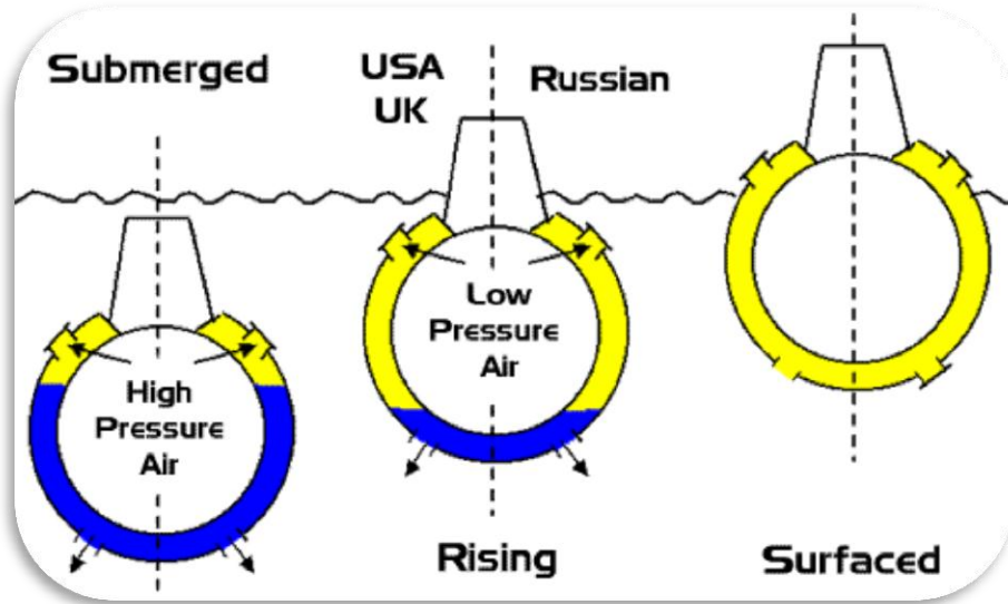
شكل (٤٢) من اليسار الى اليمين يوضح الشكل مراحل العموم بكلتا الطريقتين الروسية والغربية.
