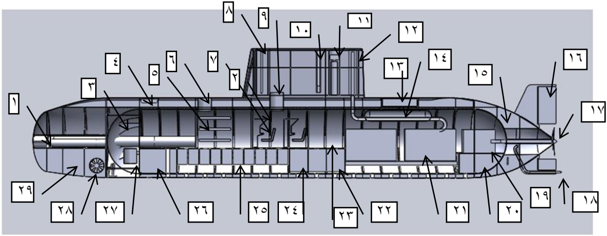
شكل (٦٢) أجزاء الغواصة من الداخل
