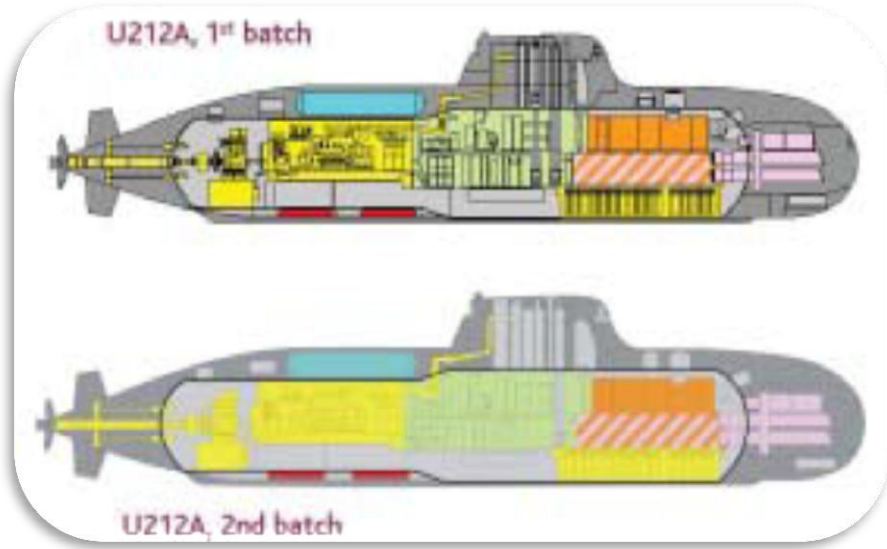
شكل (٣٦) مخطط للغواصة الألمانية Type 212 بنوعها.
