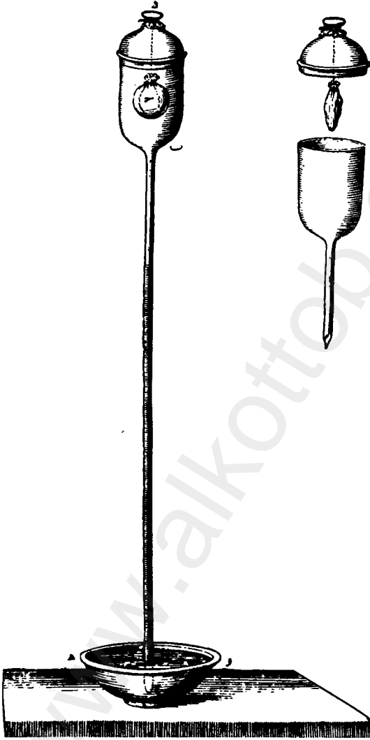
(شكل ٩) جهاز تجربة قامت بها أكاديمية التجريب « في فلورنسا . وهي ترينا كيف تتمدد المثانة، أو كيس قابل للتمدد مثلها، إذا هي وضعت في فراغ تورثشيل .
