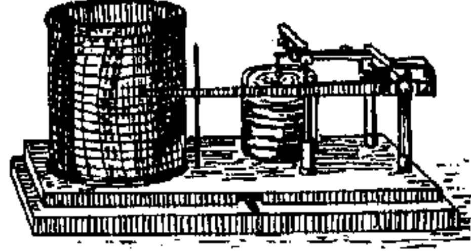
مرسمة الضّغط
