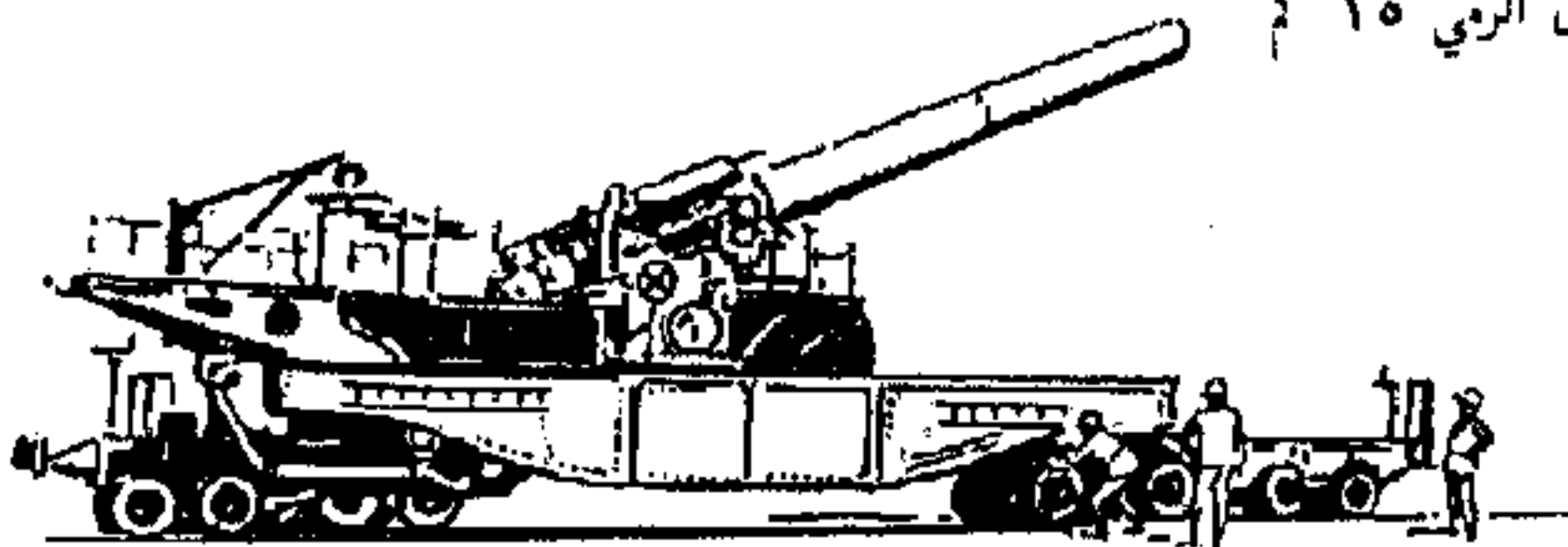
مدفع قطاري عيار ٤٠٠ ميليمتر - اختراع سنة ١٩١٨ - مدى الرمي بين ٢٥ و ٣٠ كم
