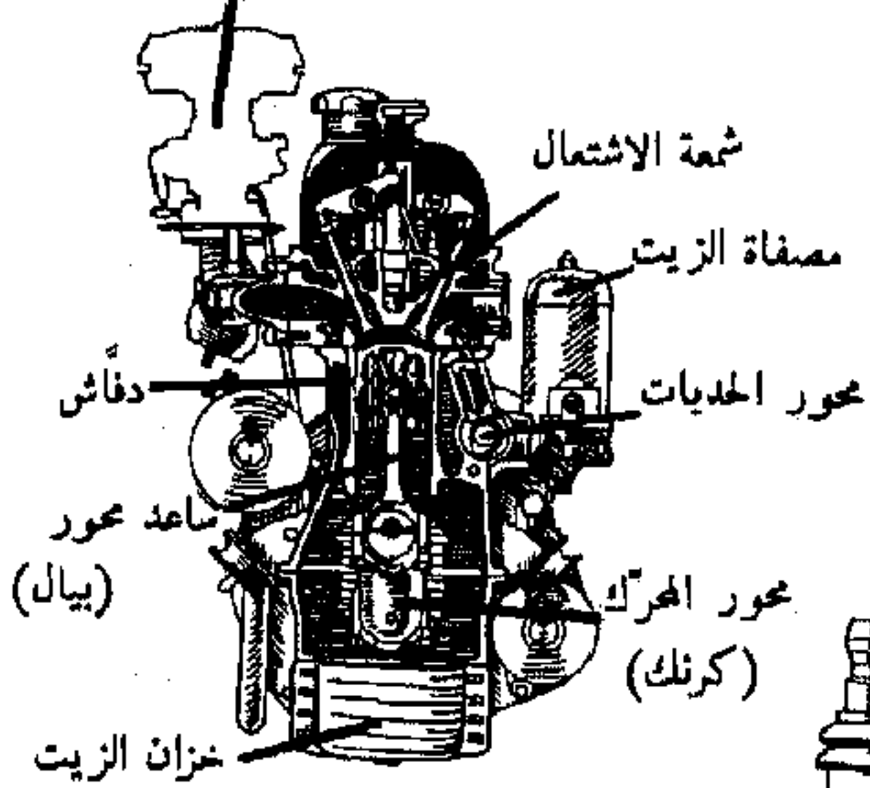
محرك : تصميم عمودي
