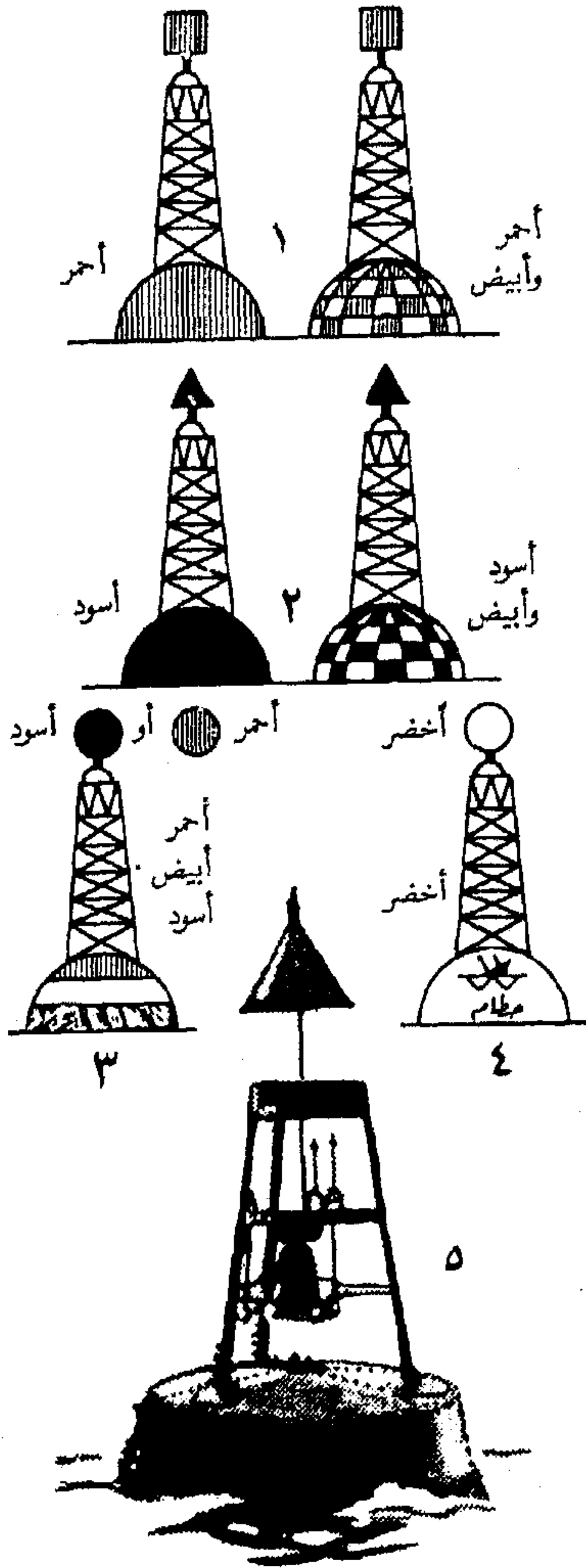
1 - ميرة سفينة. 2 - ميمنة سفينة. 3 - خطر معزولة. 4 - عظام بحرية. 5 - عوامات لها جرس 6 - عوامات مضيئة غلوة الفانر ، للإرشاد .
